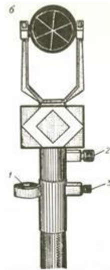
Рисунок 5 - Веха с призмным отражателем
